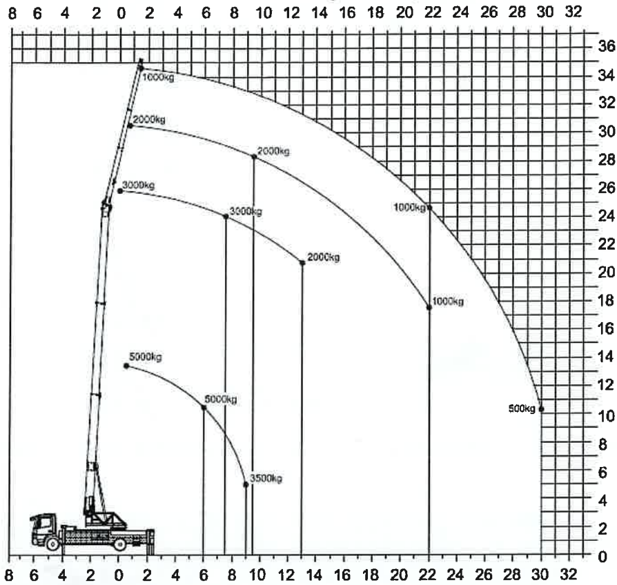
Abb. Arbeitsbereich Kranbetrieb K31-35 TSF (Traglastdiagramm)
