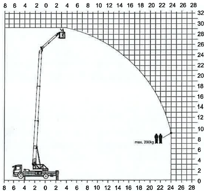
Abb. Arbeitsbereich Hubarbeitsbühnenbetrieb K31-35 TSF
